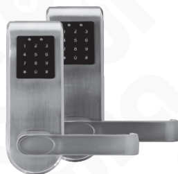
Rys 3. ELH-82B9 brass/silver szyld zamka z klawiaturą dotykową, modulem Bluetooth i czytnikiem breloków Mifare
