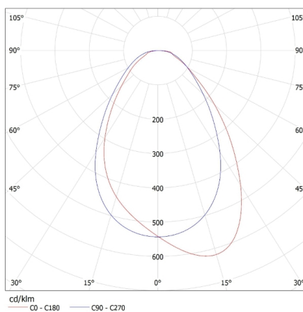
KANLUX S.A. (kat 28550) BRAVO PU36W12030NW W / LDC (Polar)
