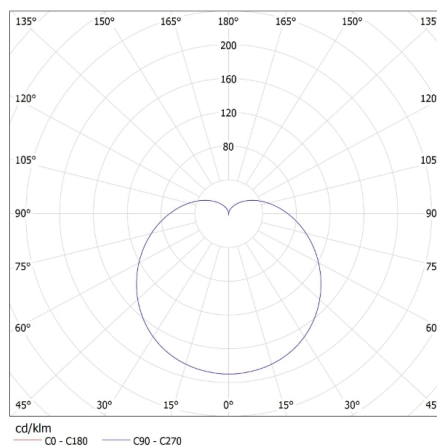
KANLUX S.A. (kat 25402) RAPID HI LED B22-WW / LDC (Polar)
