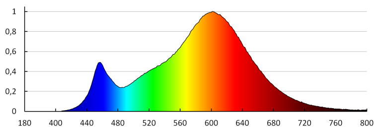
KANLUX S.A. (kat 25402) RAPID HI LED B22-WW / LDC (Polar)
